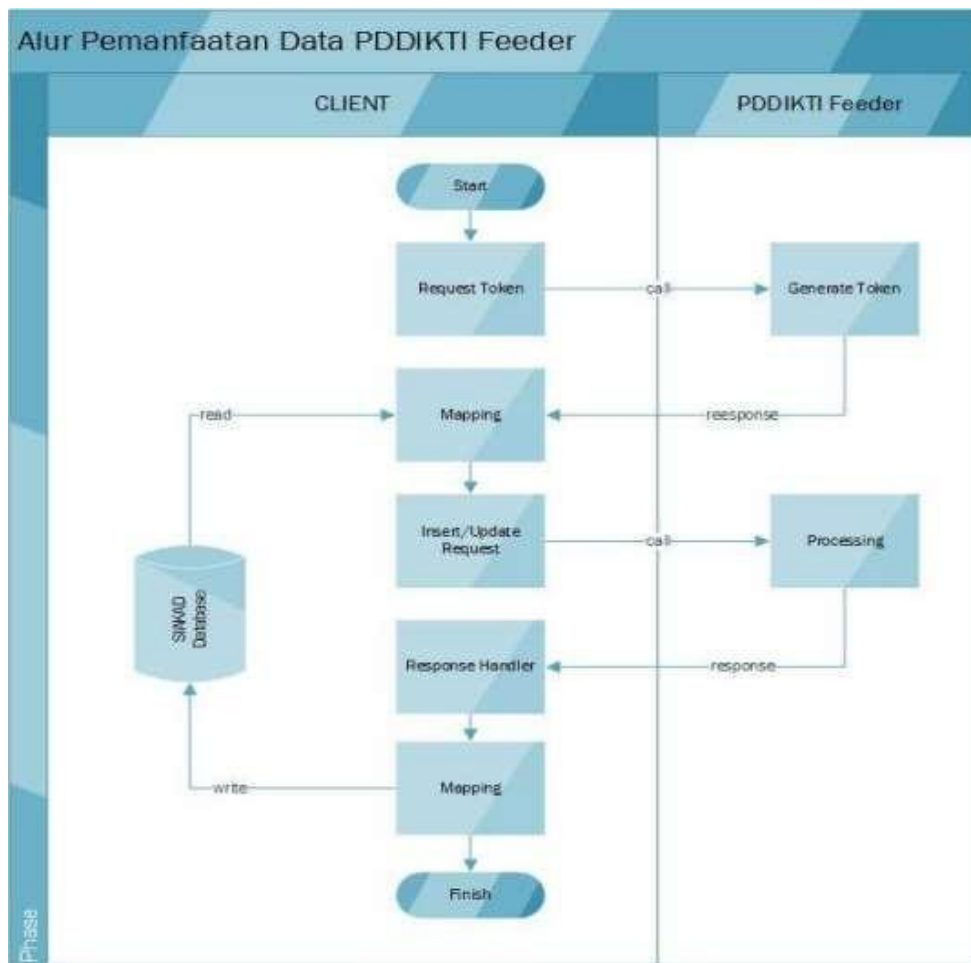
Gambar 2.2 Alur Pemanfaatan Data PDDIKTI
